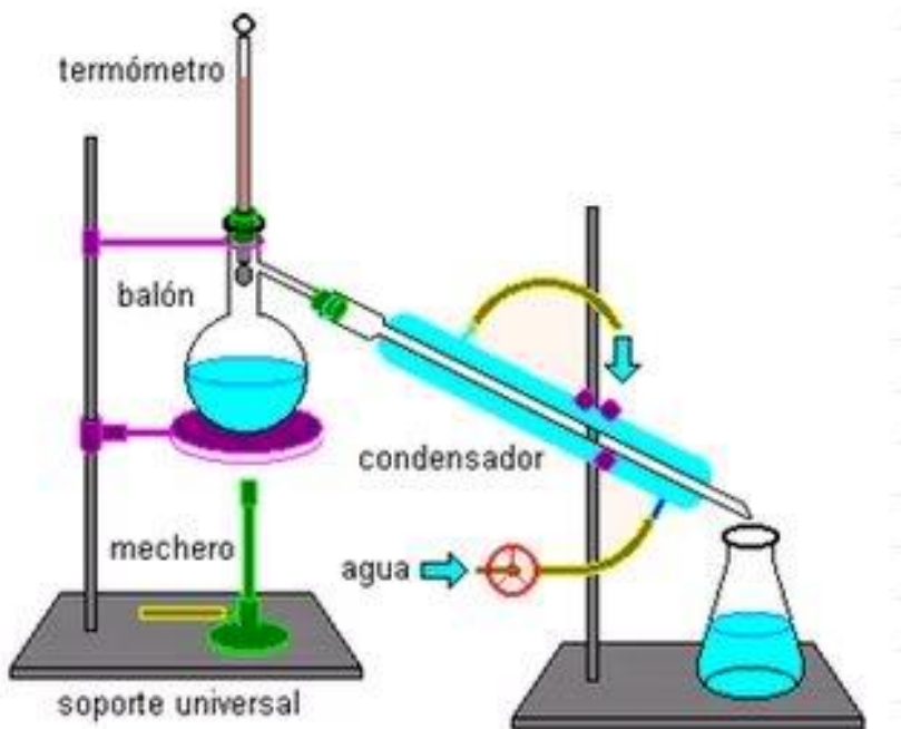
Figura 4: Destilación simple
