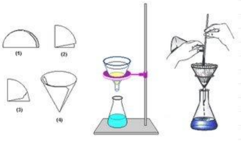
Figura 5: Filtración
